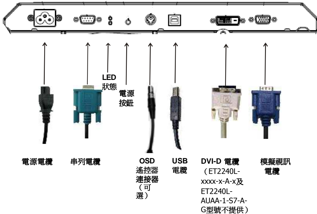
顯示器背面的連接器面板
