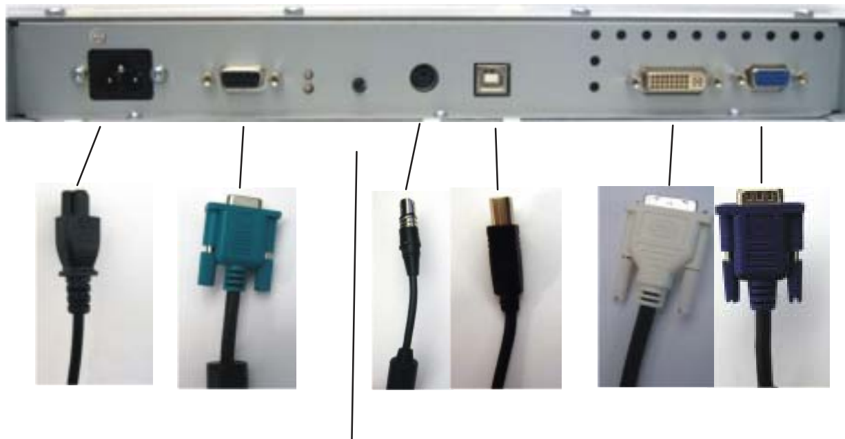
モニタ裏面のコネクタパネル
