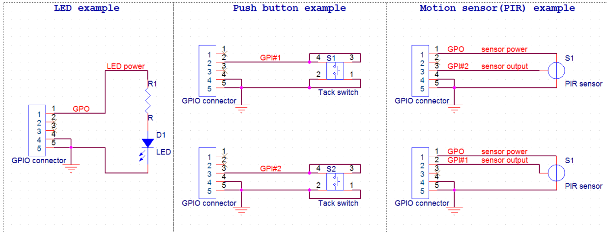
Circuit d'exemple
