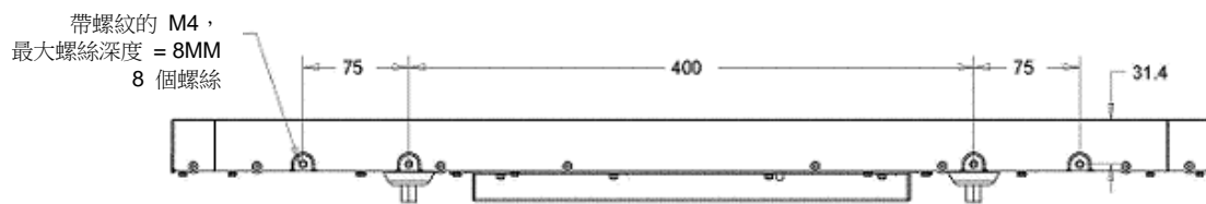
側裝橫向 (頂部/底部)
