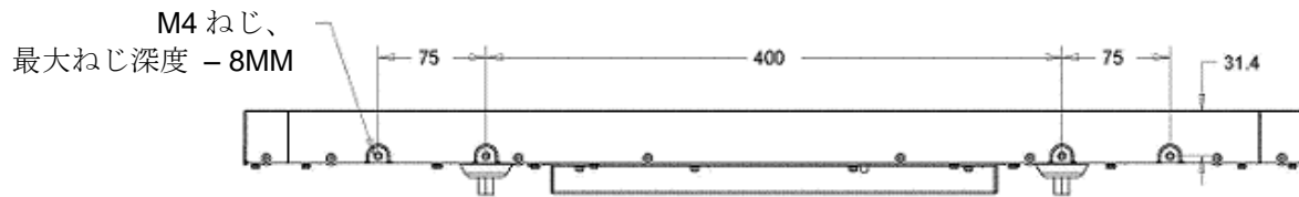
側面取り付け水平断面図 (上/下)
