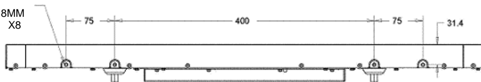
SUPPORT LATÉRAL HORIZONTAL (HAUT/BAS)
