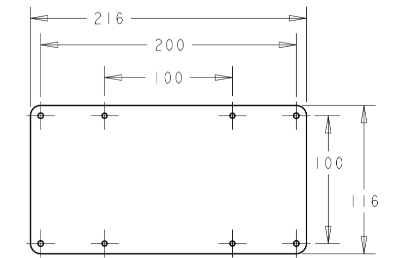
VESA MOUNT PN: E499129 SCALE 1:3
