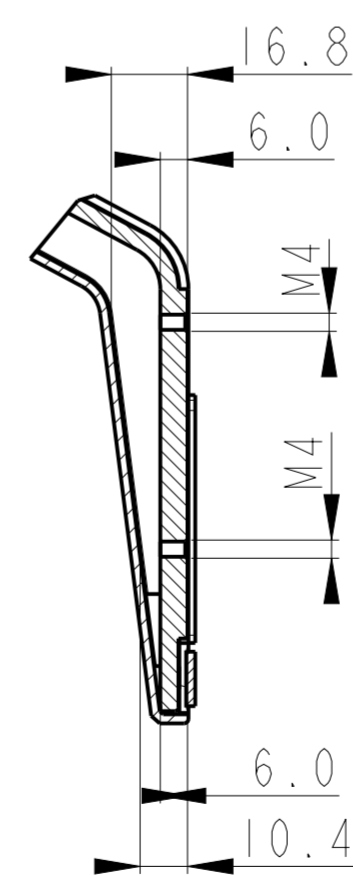
SECTION V-V
